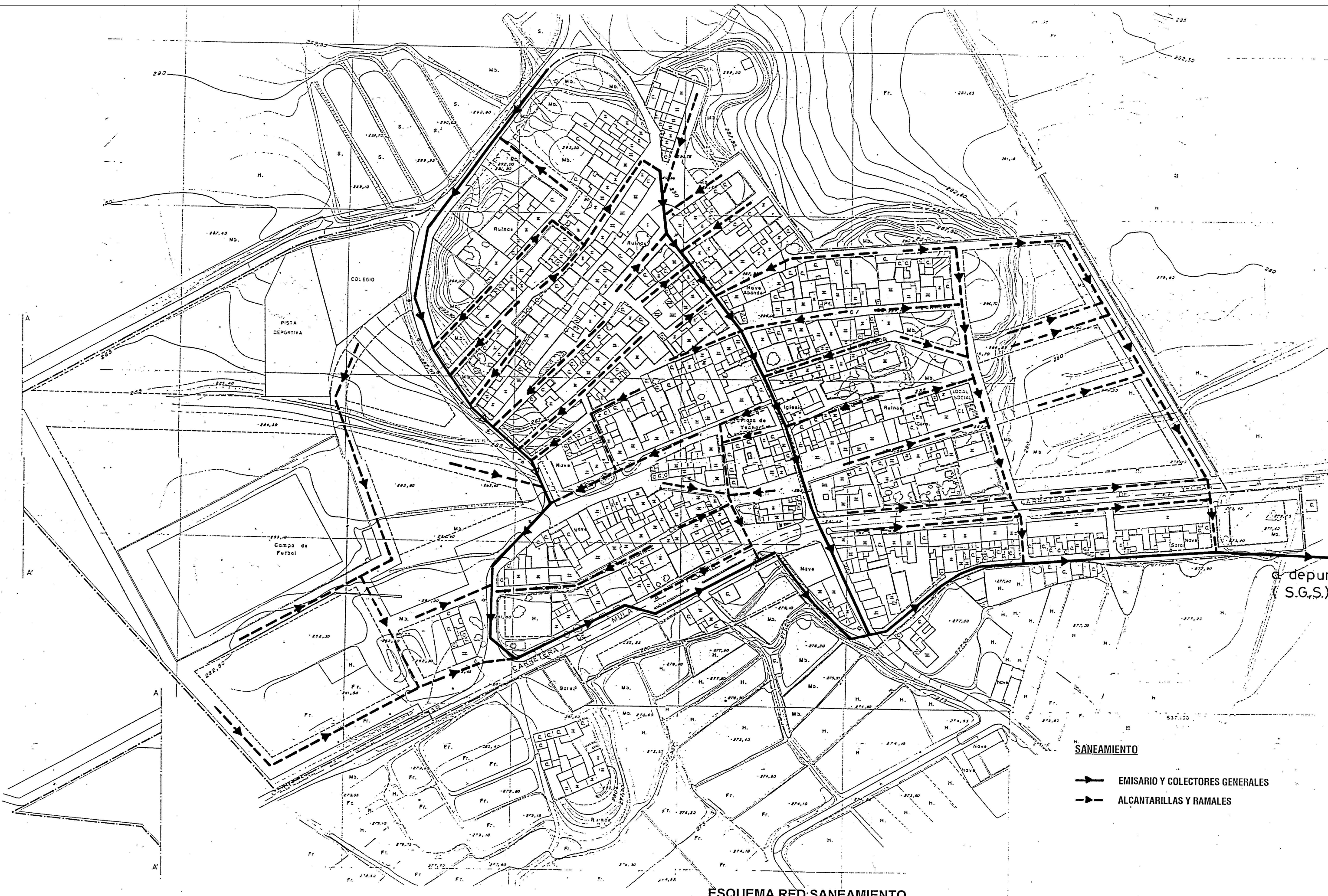
ESQUEMA RED SANEAMIENTO YECHAR
