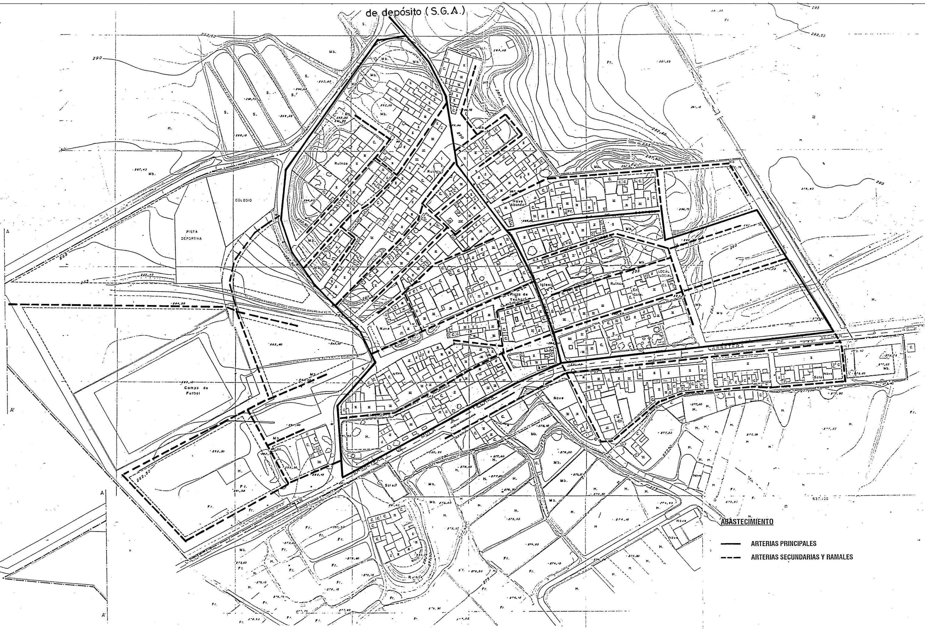
ESQUEMA RED ABASTECIMIENTO YECHAR
