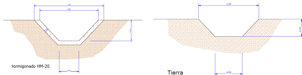
Detalle de red de Drenajes Principales y Secundarios.
