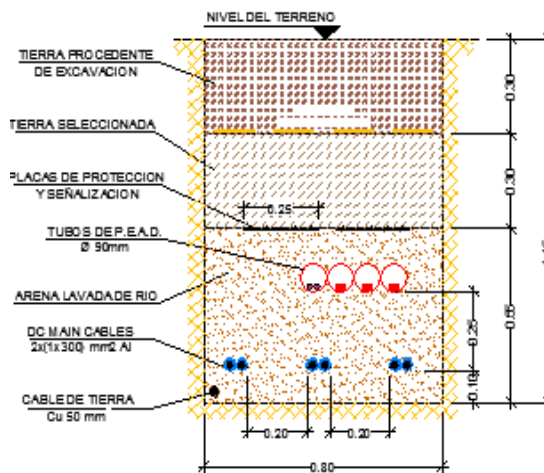
ZANJA TIPO DC2 RED BT (E: 1/20).
